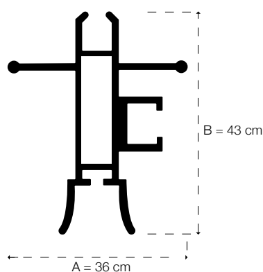
BARRAMANIGLIA PER CATENACCI
