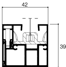
GUIDA ZIP
