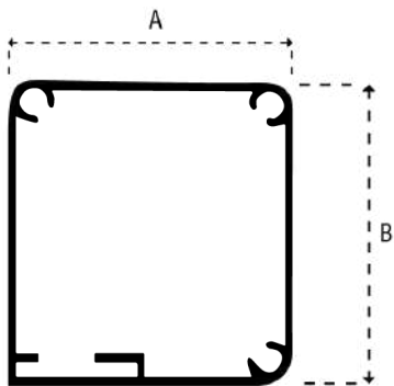
CASSONETTO A = 45 B = 51,5
