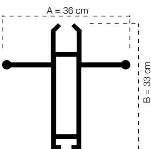
BARRAMANIGLIA
