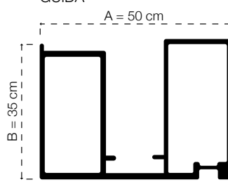
BARRAMANIGLIA PER CATENACCI
