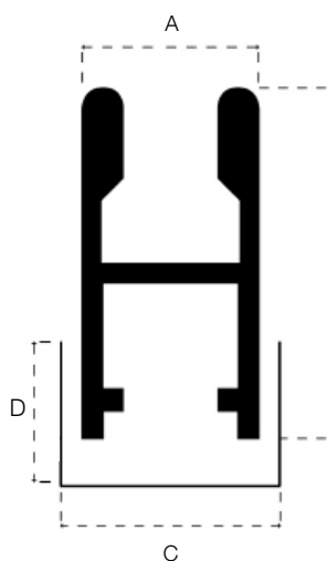
TELAIO 2 VIE
