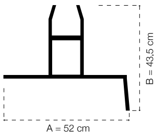
STAFFA DI FISSAGGIO
