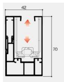
Guida maggiorata
